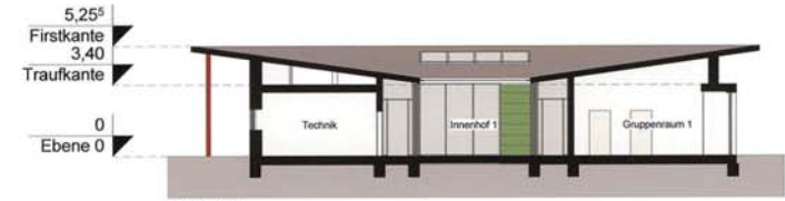
Schnitt A-A
